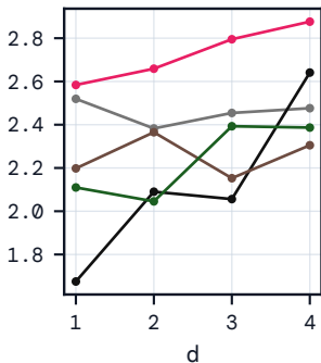
MAE (%)
